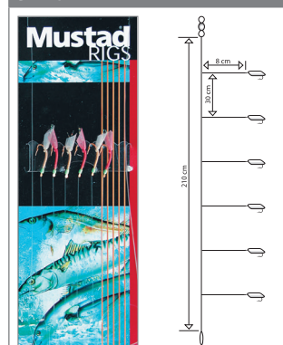
MINI SHRIMPS RIG T87 SIZE 6
